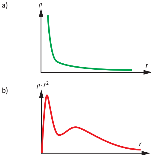
Abb. 11.1 (a) Aufenthaltswahrscheinlichkeitsdichter als Funktion des Abstands vom Atomkern; (b) Aufenthaltswahrscheinlichkeit pro Radius-Intervall
