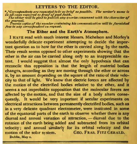
Abb. 4.3 Prärelativistische Vorstellung zur Längenkontraktion
