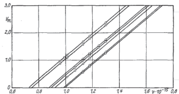
Fig. 10. Die Geraden entsprechen den Metallen (von links gerechnet): Al, Zn, Sn, Ni, Cd, Cu, Pt.
