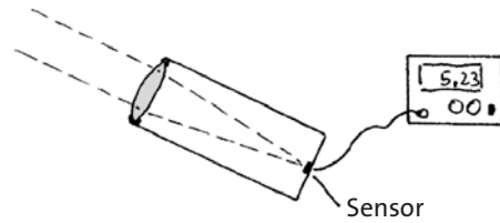
Abb. 8.11 Strahldichtemessgerät. Es misst die Strahldichte am Ort des Linseneingangs und der Richtung der optischen Achse des Geräts.
