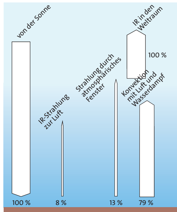
Abb. 5.11 Der Netto-Infrarot-Energiestrom durch die Atmosphäre ist klein gegen den Strom des konvektiven Wärmetransports.
